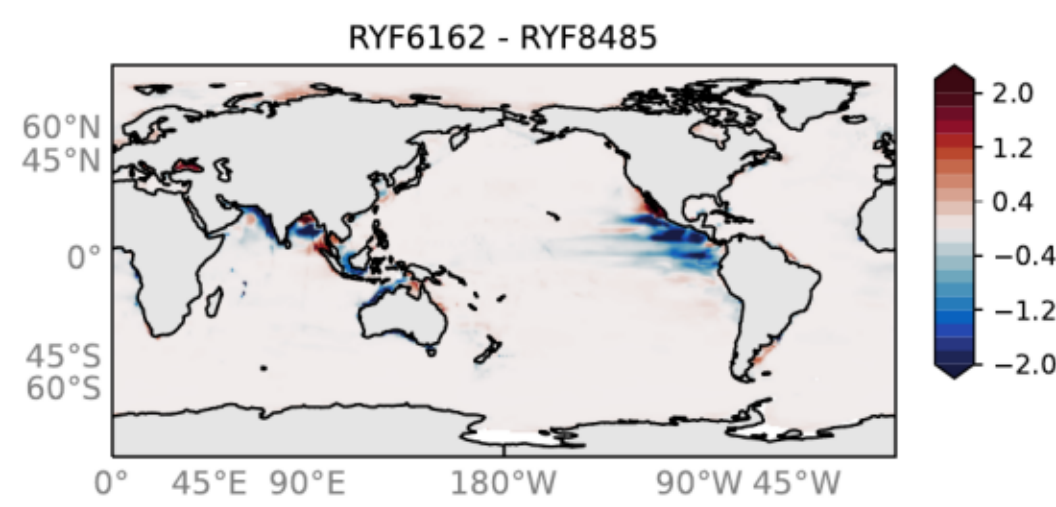
RYF6162 - RYF8485 TOC (wt-%)
